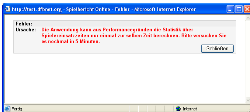
Abbildung 10: Abrufserialisierung
